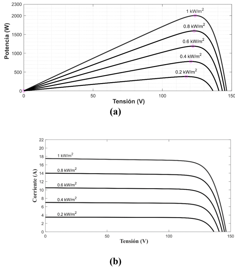
Figura 3 Curvas características I-V (a) y P-V (b) ante la variación de la irradiancia.
