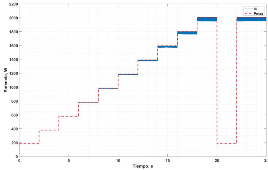
Figura 14 Simulación del MPPT con IC.
