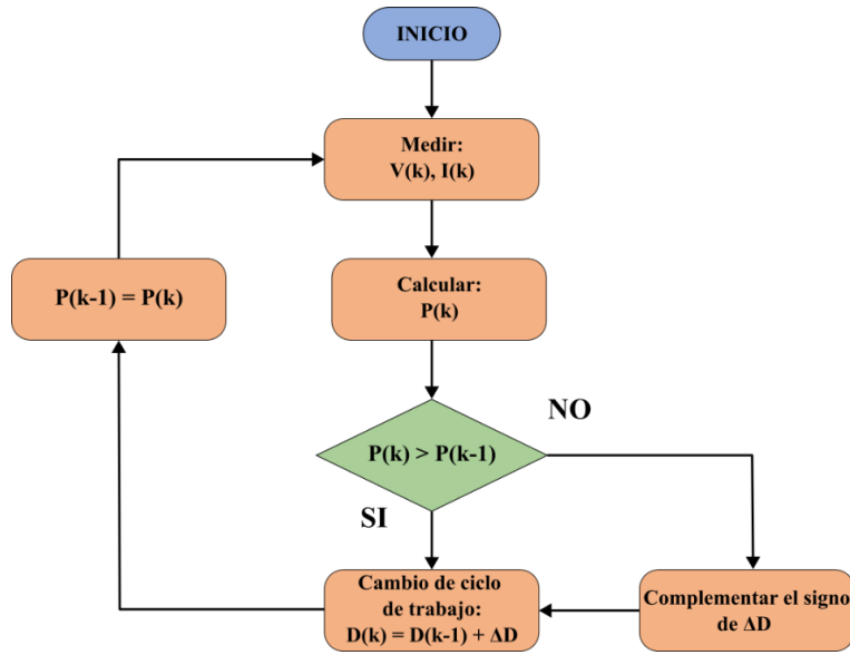
Figura 6 Diagrama de flujo de Escalada de Colina (HC)
