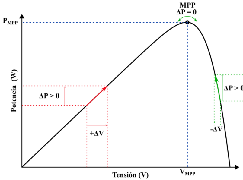
Figura 4 Técnica MPPT convencional P&O
