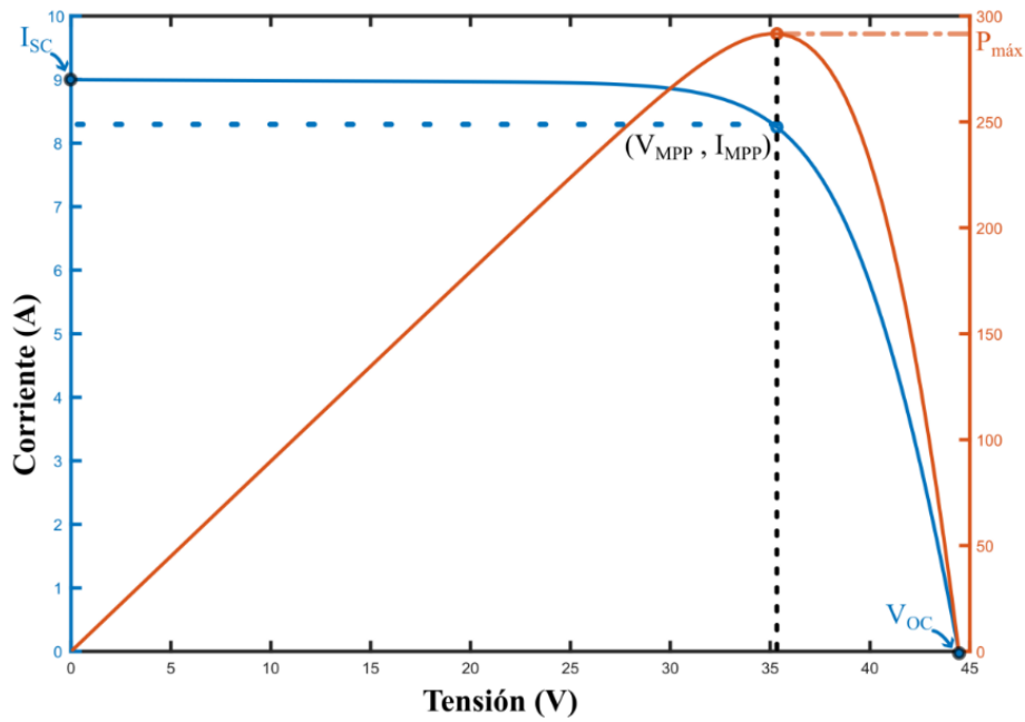
Figura 2 Curvas características I-V y P-V.
